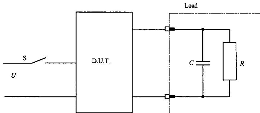
a) 启动过程中的电流测量线路
