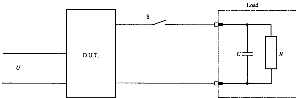
a) 启动过程中的电流测量线路
