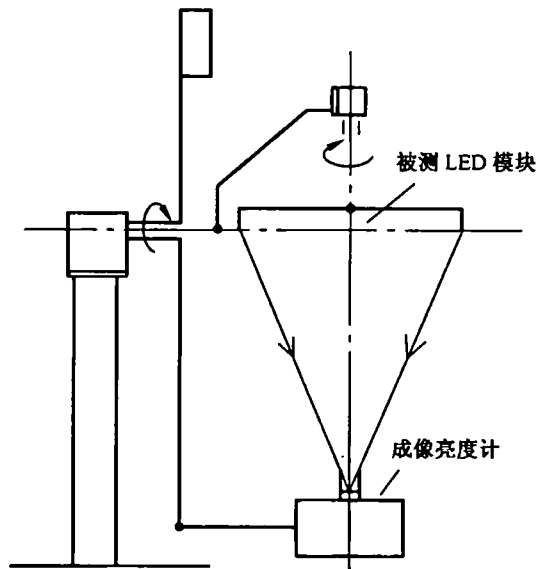
图 A.7 近场分布光度计
