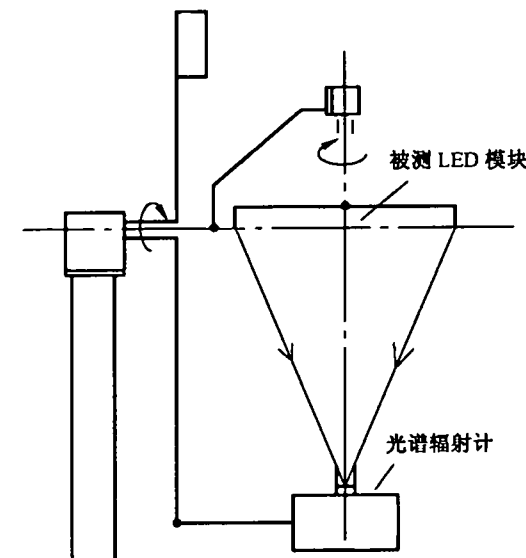
图 A.6 典型分布光谱辐射计示意图
