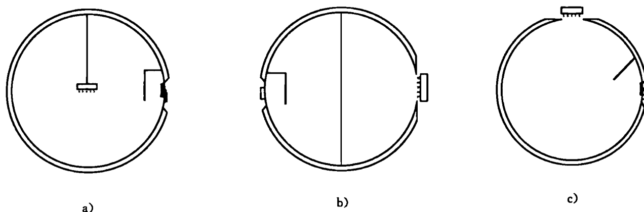
图 3 积分球测量示意图
