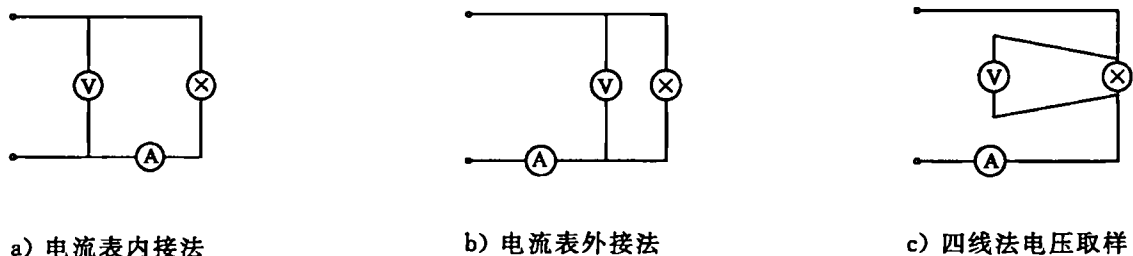
图 1 电性能测量示意图
