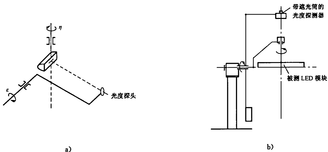
图 A.1 CIE 84 推荐的测量光通量的探测器旋转式分布光度计原理 a)和结构 b)示意图
