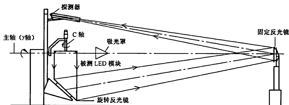
图 A.3 双镜分布光度计示意图
