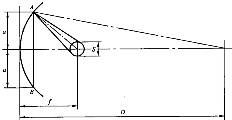
图 B.1 投光灯的最小测量距离
