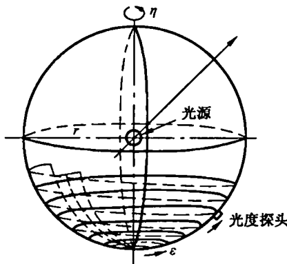
图 2 光通量的计算原理示意图
